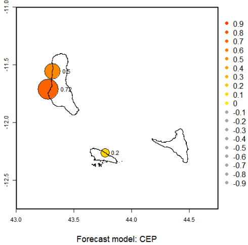
Score RPSS: RR OND-2020 It1
